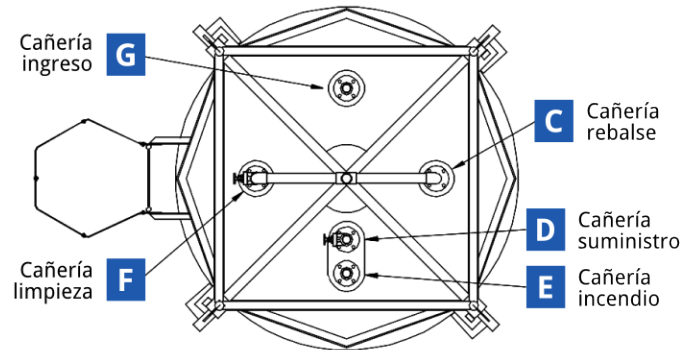
Corte A-A
